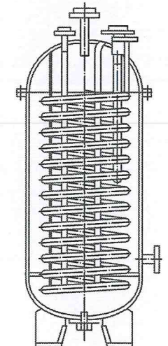
Испаритель
