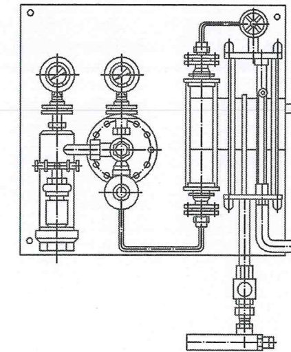
Хлоратор ЛОНИИ-100
