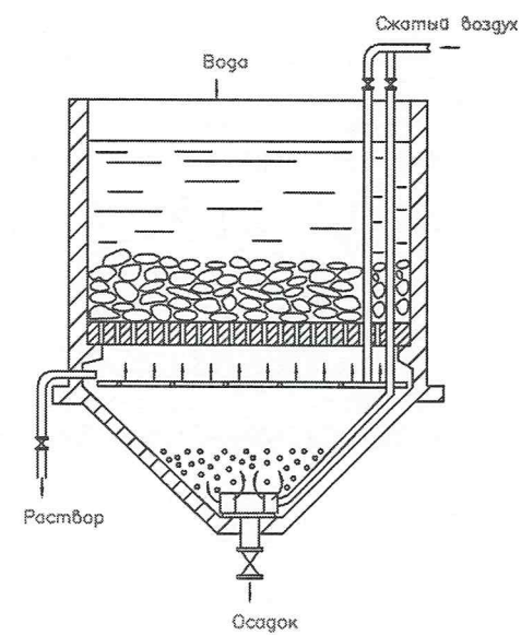
Растворный бак
