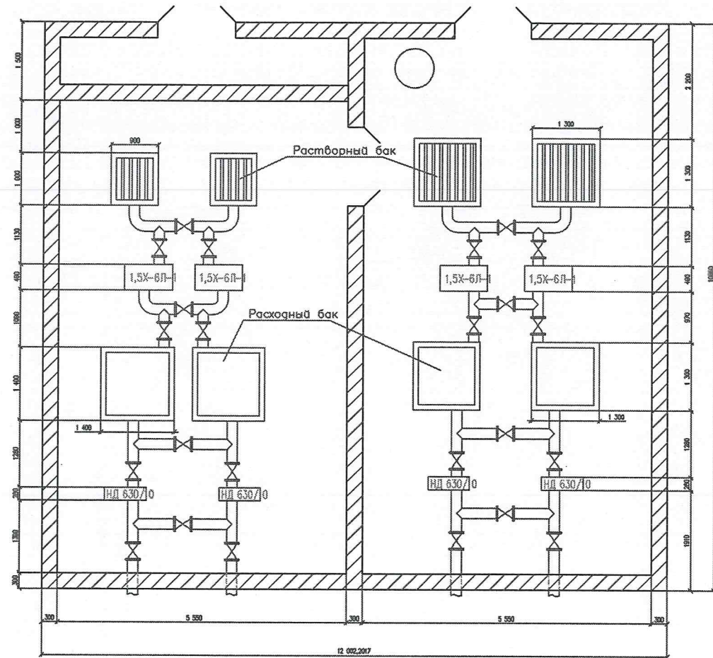
Растворный бак
