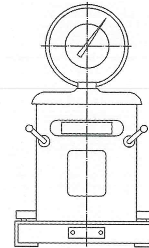
Весы
