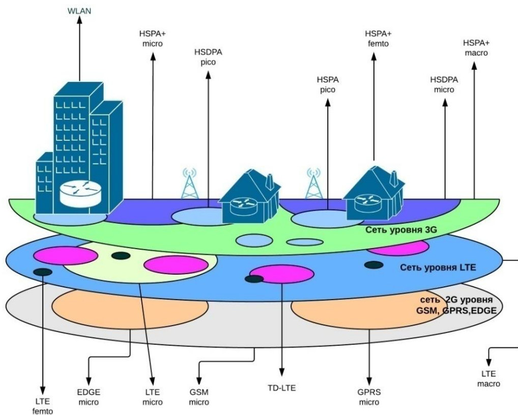
1.1 сурет – Гетерогенді сымсыз желінің сұлбасы
