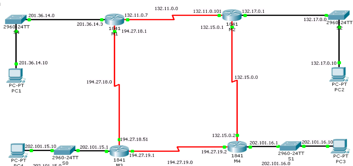
2.2-сурет - RIP роутерларынан құралған желі
