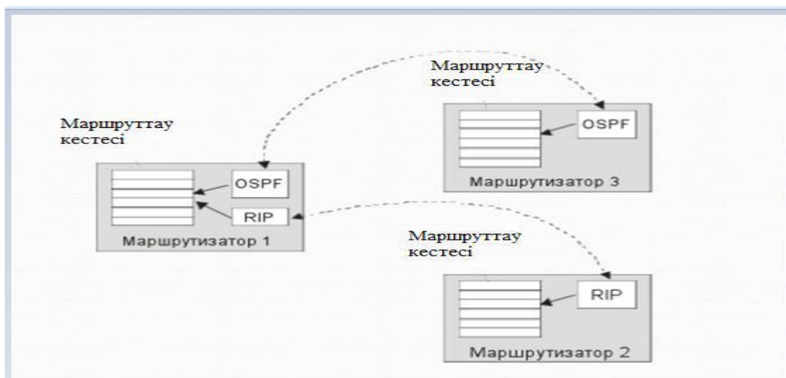
2.7 - сурет - RIP пен OSPF протоколдарының бір желіде жұмыс істеу принципі
