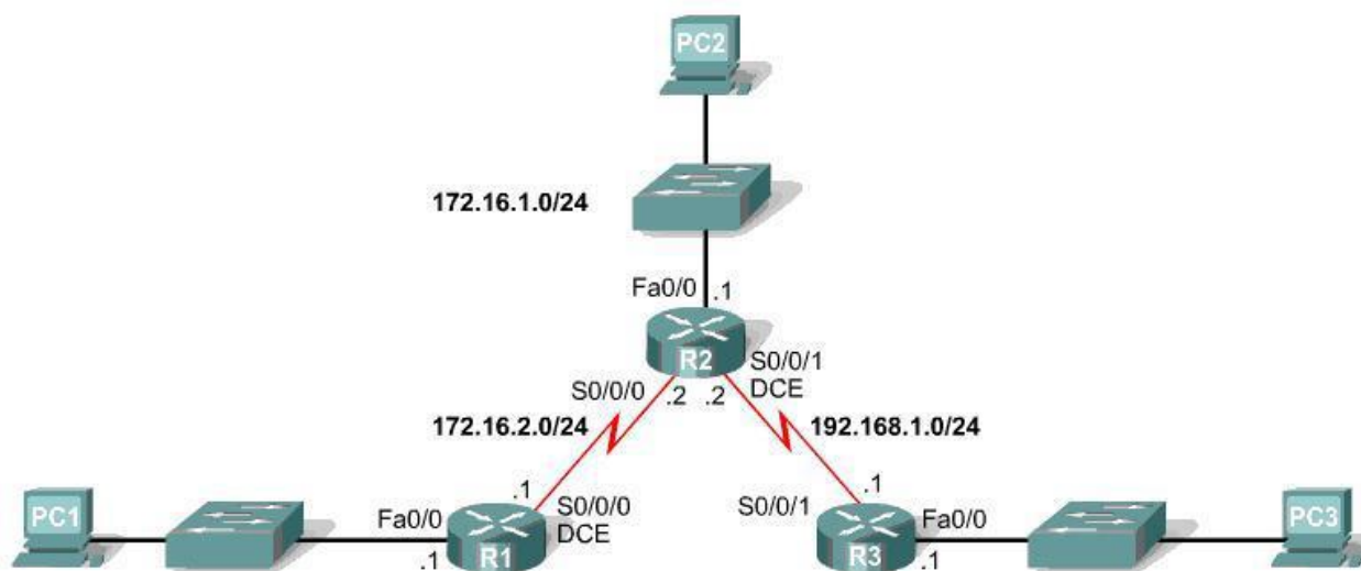
2.1-сурет - Статикалық маршруттаудың жүзеге асырылуы
