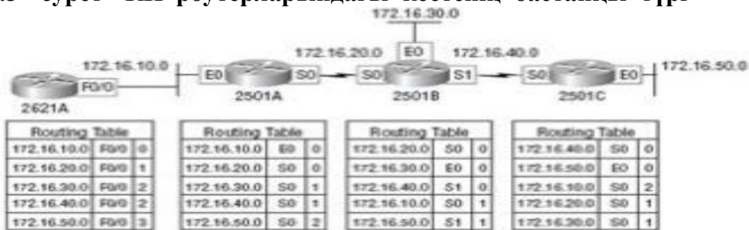
2.4 - сурет - Маршрутты ақпарат кеткеннен кейінгі кесте түрі
