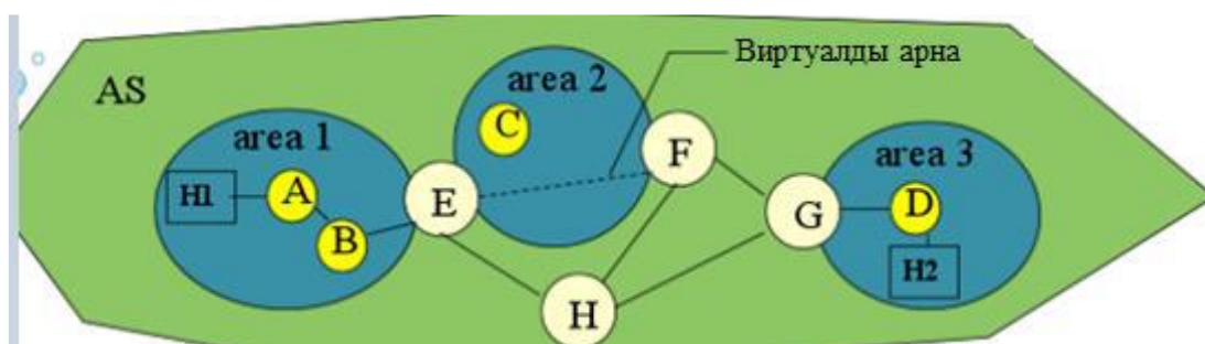
2.5 - сурет - OSPF иерархиясы
