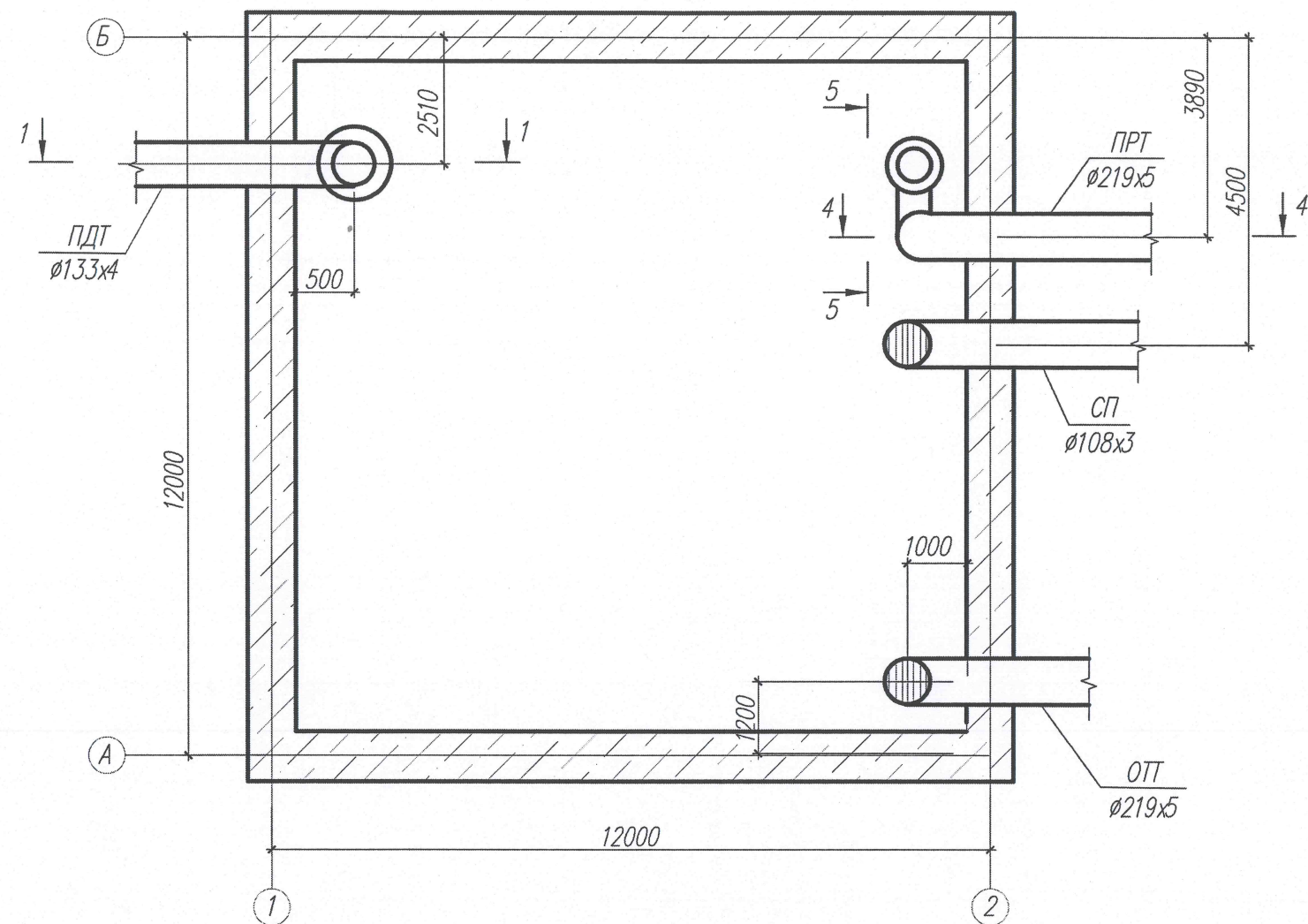
План резервуара на отметке +2,000
