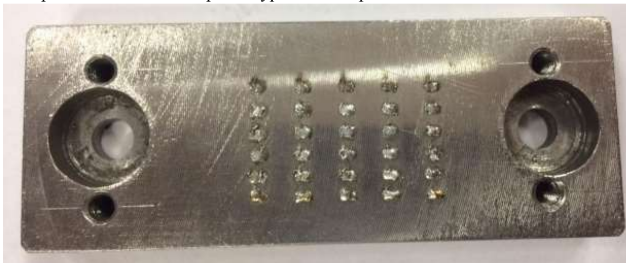
25 – сурет- Бірнеше қабатты үлгінің торы түрінде балқыту
