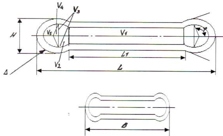
Рисунок 2.3 – Схема пневмоэлемента
