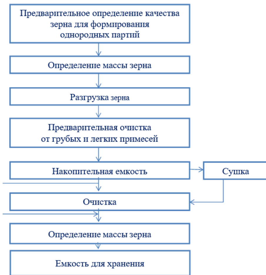
Рисунок 10 – Последовательность основных этапов технологического процесса на предприятиях по приёму, очистке, сушке и хранению зерна 1.3.3 Аспирация элеваторов, конвейеров, зерносушилок, зернохранилищ
