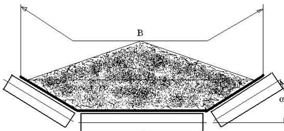
Рисунок 11– Профиль поперечного слоя транспортируемого материала при использовании желобчатых роликоопор.
