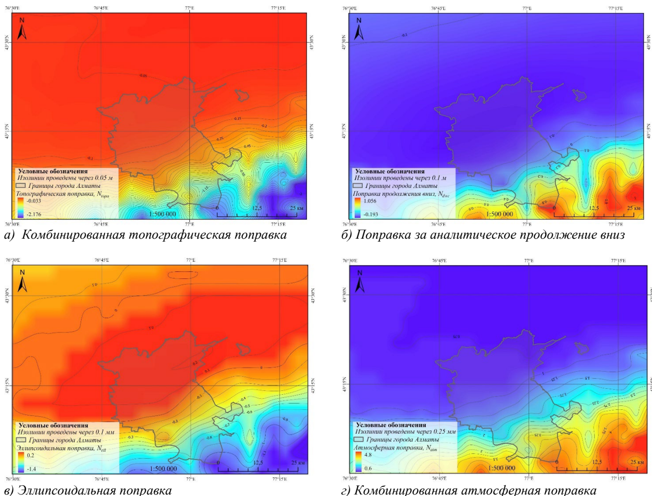
Рисунок 5.2.4 - Поправки к приблизительным высотам геоида с использованием
