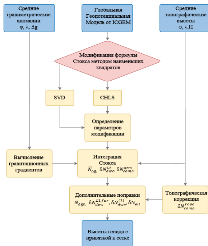
Рисунок 5.2.1 - Блок-схема алгоритма вычисления [104]
