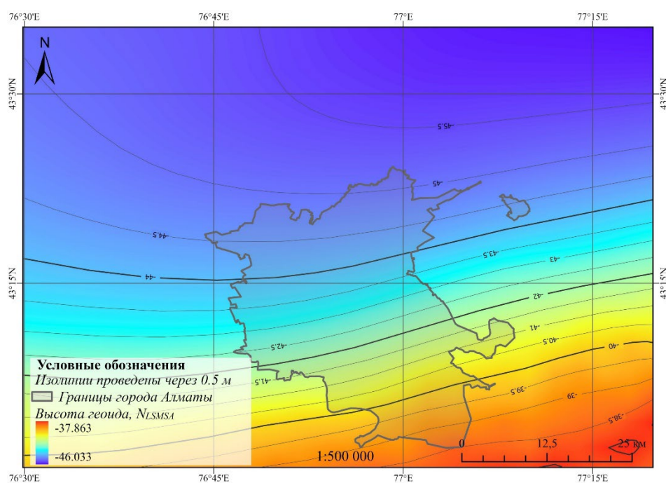
Рисунок 5.2.5 – Высота геоида по методу Модификации формулы Стокса методом наименьших квадратов N_{LSMS} , м
