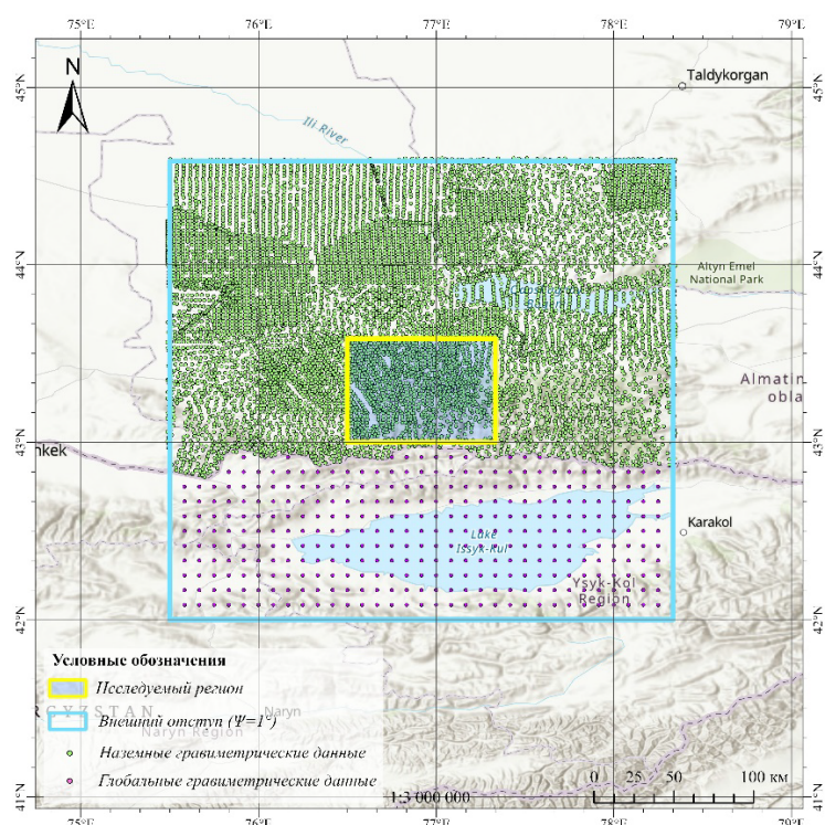
Рисунок 3.6.2 – Комбинирование наземных гравиметрических данных с глобальными
