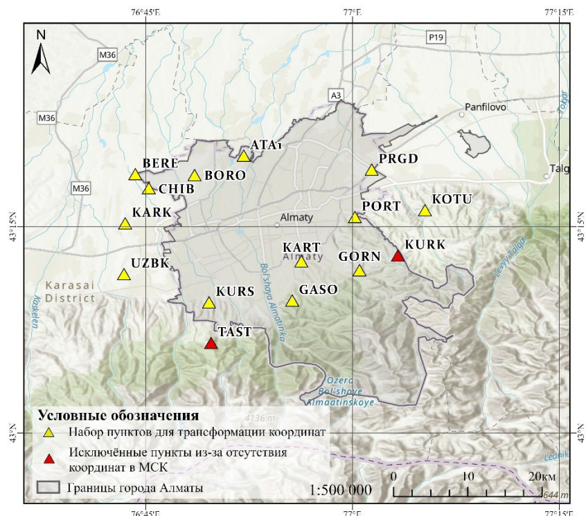
Рисунок 4.1. - Схема расположения геодезических пунктов, участвующих в трансформации координат
