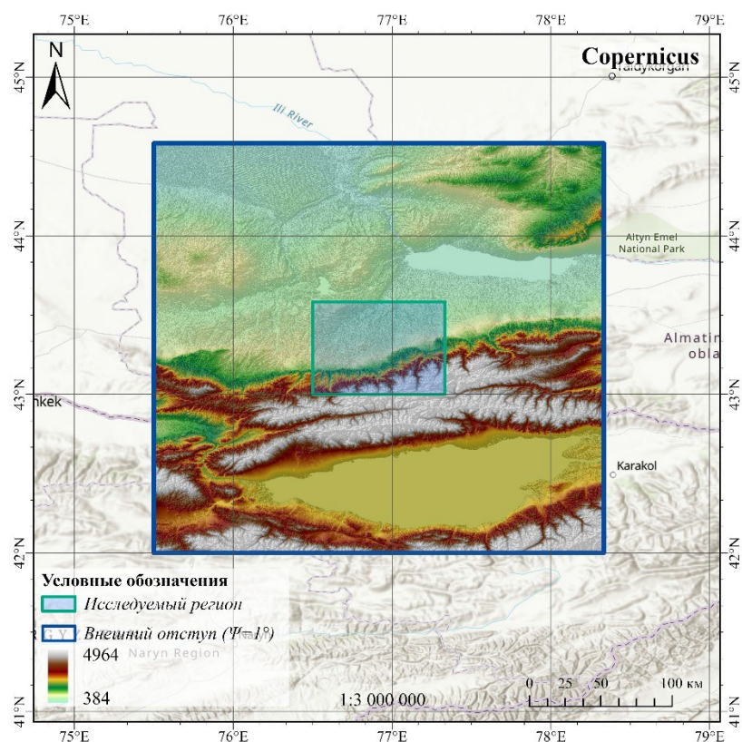
Рисунок 3.7.3 – Цифровая модель рельефа Copernicus
