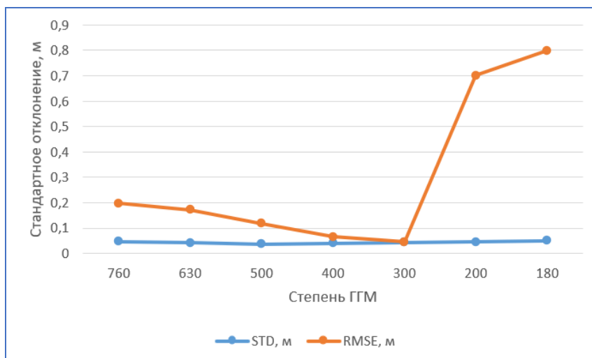
Рисунок 5.2.2 - График изменения статистики с уменьшением степени ГГМ с дисперсией ошибок наземных гравиметрических данных C(0)=1 \text{ мГал}^2
