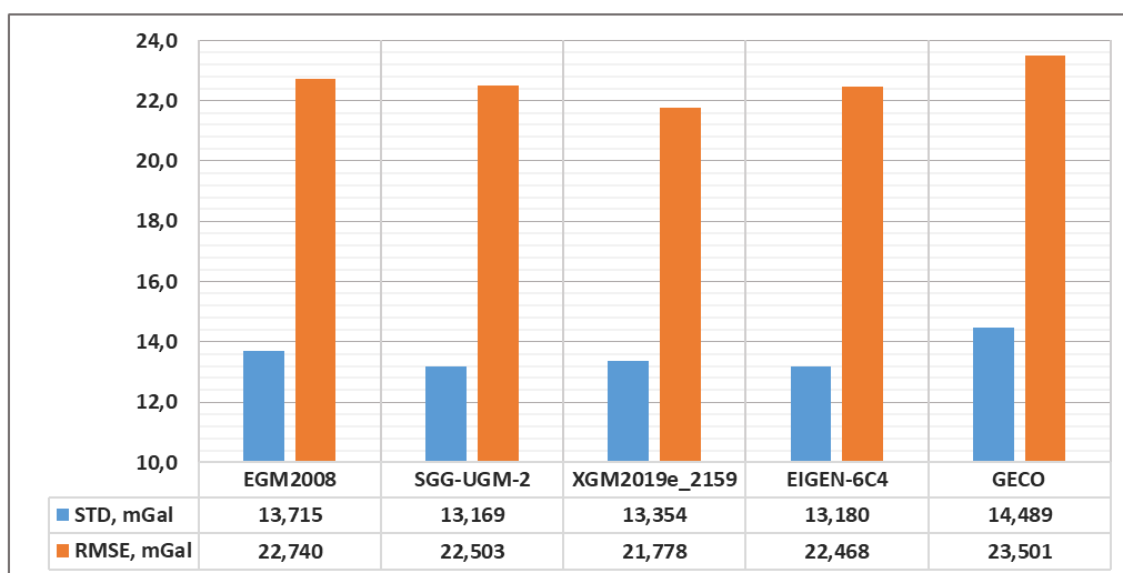
Рисунок 3.8.2 - Сравнение стандартного отклонения (STD) и среднеквадратичного отклонения (RMSE) между значениями аномалий Буге по различным ГГМ и наземными наблюдениями
