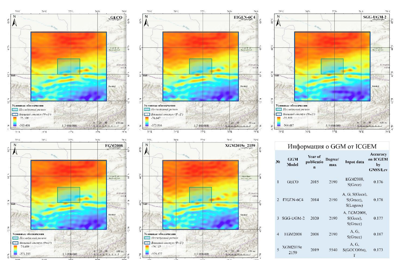
Рисунок 3.8.1 – Значения аномалии Буге отобранных Глобальных геопотенциальных моделей
