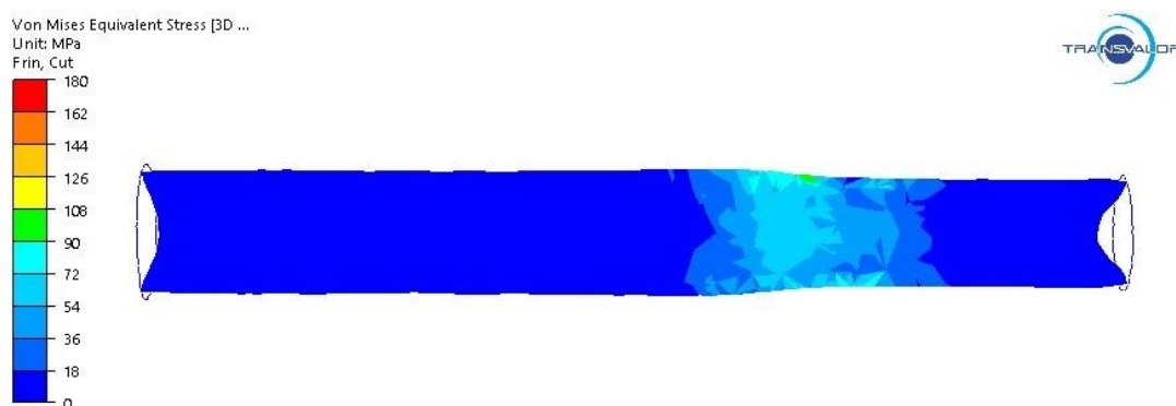
Сурет 3.34 – Радиалды-ығыстыра илемдеудің екінші өтімінен кейінгі (40–35 мм) шыбықтың бойлық қимасындағы эквивалентті кернеулер мәндерінің таралуы
