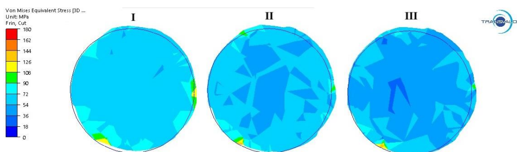
Сурет 3.32 – Радиалды-ығыстыра илемдеудің бірінші өтімінен кейінгі (45–40 мм) шыбықтың ұзындығы бойынша әртүрлі учаскелеріндегі көлденең қималарда эквивалентті кернеулер мәндерінің таралуы (I – шыбықтың басы; II – ортасы; III – соңы)
