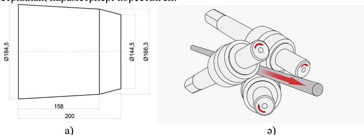
Сурет 2.2 – Біліктердің геометриялық параметрлері (а) және олардың илемдеу орнағынаң жұмыс аймағындағы орналасуы (ә)
