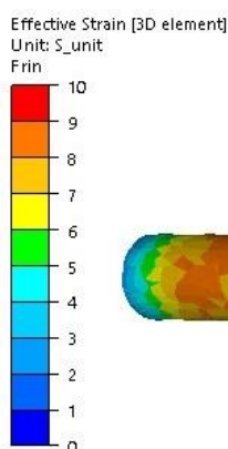
Сурет 3.27 – Радиалды-ығыстыра илемдеудің үшінші өтімінен кейінгі (35–30 мм) шыбық беті бойынша пластикалық деформация интенсивтілігінің кеңістіктік таралуы
