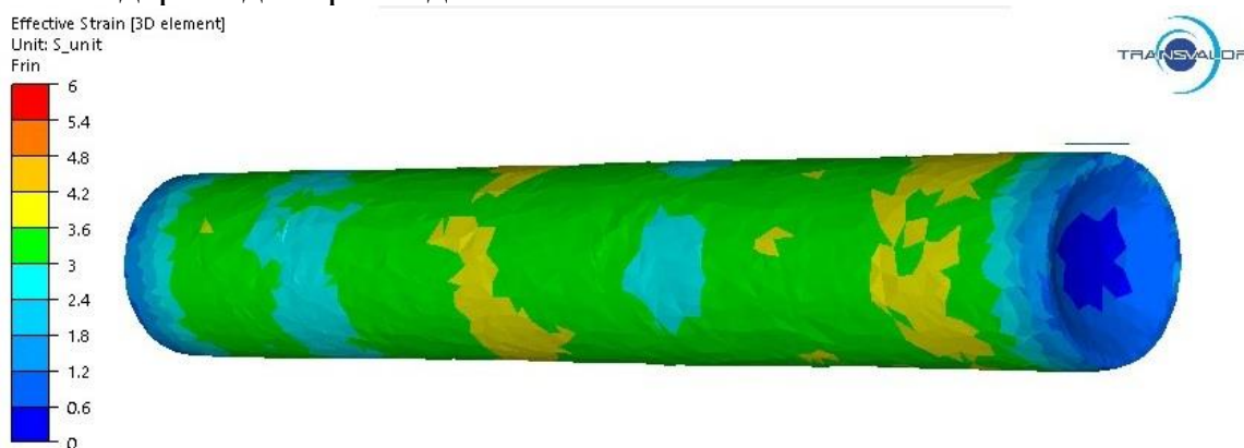
Сурет 3.21 – Радиалды-ығыстыра илемдеудің бірінші өтімінен кейінгі (45–40 мм) шыбық беті бойынша пластикалық деформация интенсивтілігінің кеңістіктік таралуы
