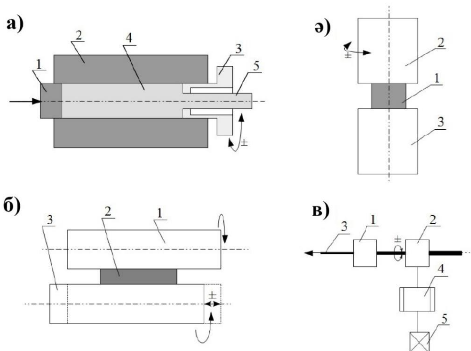
Сурет 1.4 – КОВО әдісі бойынша металл материалдарын пластикалық деформациялау үдерістерінің техникалық шешімдерінің мысалдары [66]: а) престоу (1 – пуансон, 2 – контейнер, 3 – қосжақты айналмалы матрица, 4 – металл дайындама, 5 – алынатын бұйым); ә) соғу (1 – металл дайындама, 2 – қосжақты айналмалы пуансон, 3 – матрица); б) илемдеу (1 – металл дайындама, 2 – үстіңгі білік, 3 – циклдік осьтік ығысумен төменгі білік); в) созу (1 – қозғалмайтын білік, 2 – қосжақты айналмалы білік, 3 – металл дайындама, 4 – беріліс қорабы, 5 – жетек қозғалтқыш).
