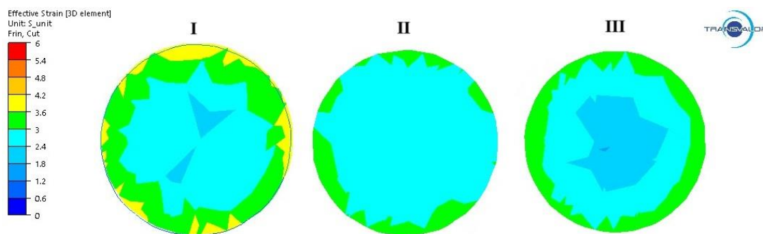
Сурет 3.23 – Радиалды-ығыстыра илемдеудің бірінші өтімінен кейінгі (45–40 мм) шыбықтың ұзындығы бойынша әртүрлі учаскелеріндегі көлденең қималарда пластикалық деформация интенсивтілігінің таралуы (I – шыбықтың басы; II – ортасы; III – соңы)
