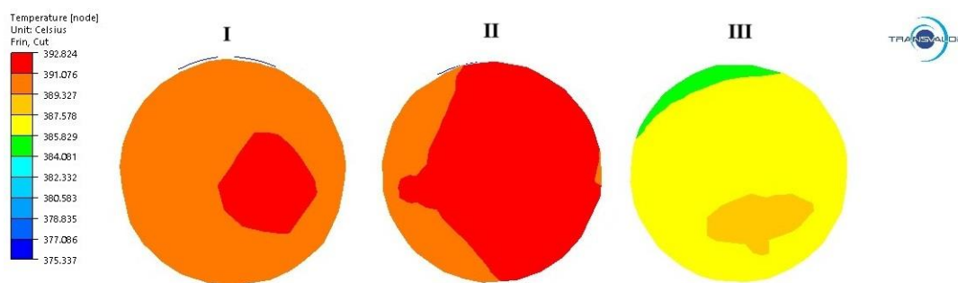
Сурет 3.17 – Радиалды-ығыстыра илемдеудің екінші өтімінен кейінгі (40–35 мм) шыбықтың ұзындығы бойынша әртүрлі учаскелеріндегі көлденең қималарда температураның таралуы (I – шыбықтың басы; II – ортасы; III – соңы)
