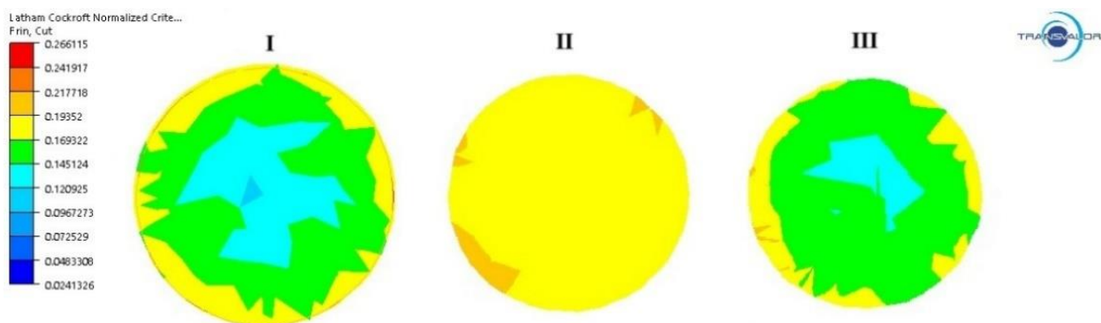
Сурет 3.41 – Радиалды-ығыстыра илемдеудің алғашқы өтуінен кейінгі (45–40 мм) шыбықтың ұзындығы бойынша әртүрлі бөліктеріндегі көлденең қималарында Лэтэм–Кокрофт бұзылу критерийі мәндерінің таралуы
