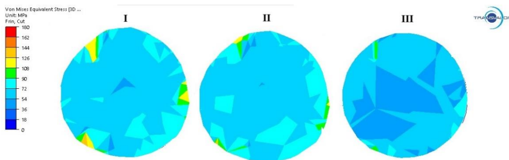
Сурет 3.34 – Радиалды-ығыстыра илемдеудің екінші өтімінен кейінгі (40–35 мм) шыбықтың бойлық қимасындағы эквивалентті кернеулер мәндерінің таралуы
