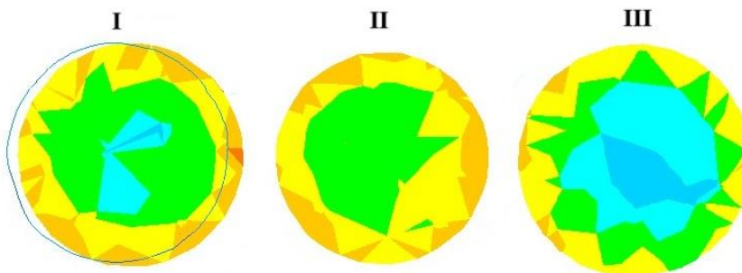
Сурет 3.26 – Радиалды-ығыстыра илемдеудің екінші өтімінен кейінгі (40–35 мм) шыбықтың ұзындығы бойынша әртүрлі учаскелеріндегі көлденең қималарда пластикалық деформация интенсивтілігінің таралуы (I – шыбықтың басы; II – ортасы; III – соңы)
