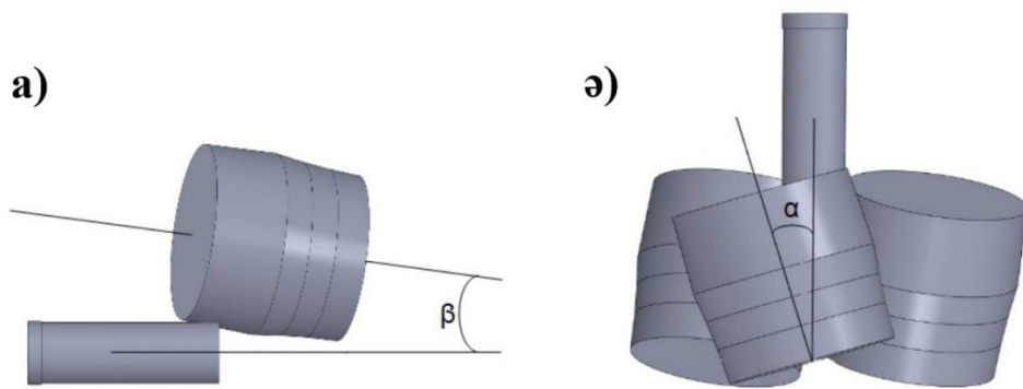
Сурет 1.6 – Үшбілікті қиғаш орнақтағы біліктердің орналасу бұрыштары: а) тік жазықтықта; ә) көлденең жазықтықта.
