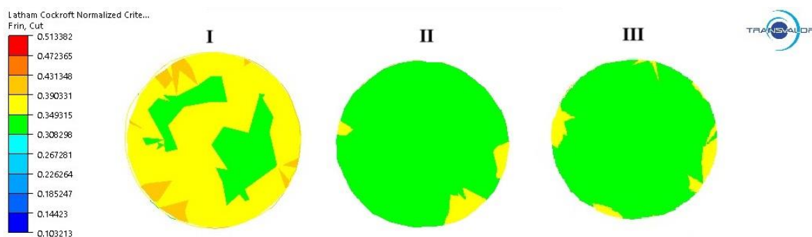
Сурет 3.43 – Радиалды-ығыстыра илемдеудің екінші өтуінен кейінгі (40–35 мм) шыбықтың бойлық қимасындағы Лэтэм–Кокрофт бұзылу критерийі мәндерінің таралуы
