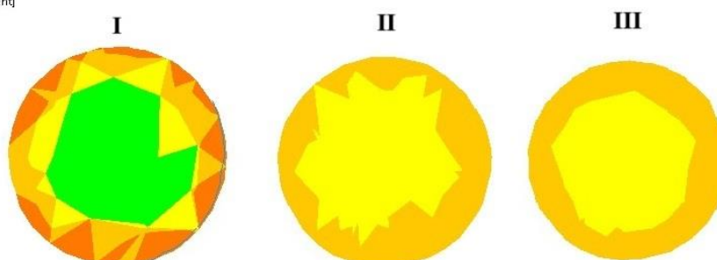
Сурет 3.29 – Радиалды-ығыстыра илемдеудің үшінші өтімінен кейінгі (35–30 мм) шыбықтың ұзындығы бойынша әртүрлі учаскелеріндегі көлденең қималарда пластикалық деформация интенсивтілігінің таралуы (I – шыбықтың басы; II – ортасы; III – соңы)
