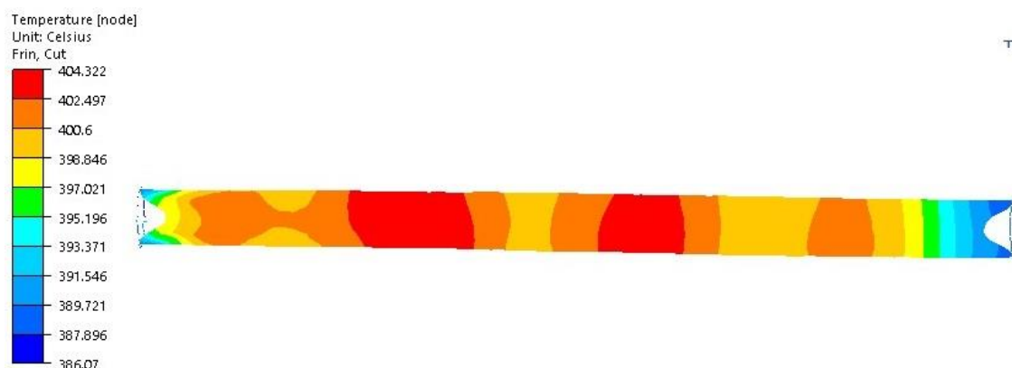
Сурет 3.19 – Радиалды-ығыстыра илемдеудің үшінші өтімінен кейінгі (35–30 мм) шыбықтың бойлық қимасындағы температураның таралуы
