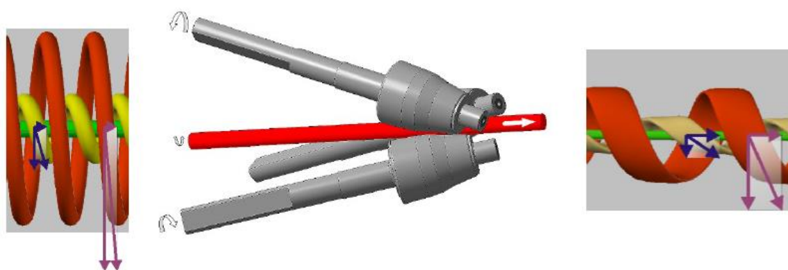
Сурет 1.5 – Радиалды-ығыстыру илемдеу сызбасы және металдың ағын сипаты: осьтік, аралық және беткі аймақтарда, илемдеу калибрінің деформациялық аймағына дейінгі және кейінгі күйі [71].
